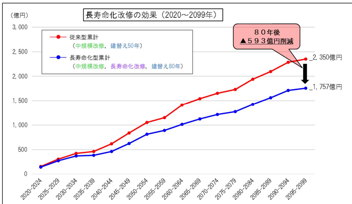
図5) 長寿命化改修による削減効果
