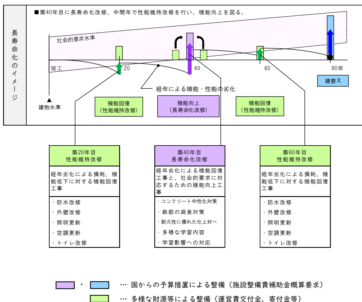
図4）長寿命化の改修サイクル（概念図）
