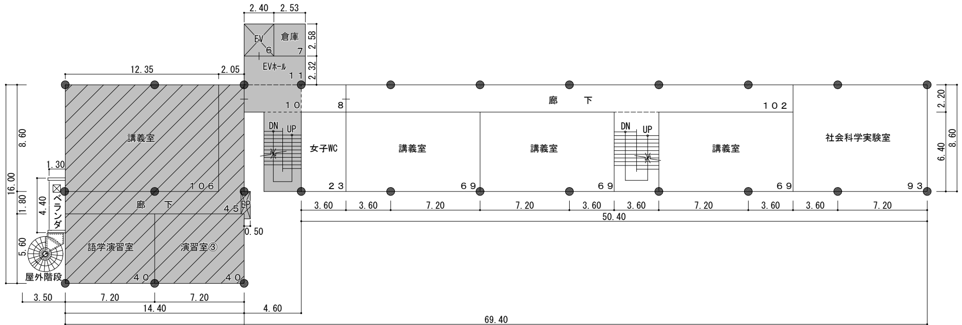
改修前 3階平面図 S=1/300
