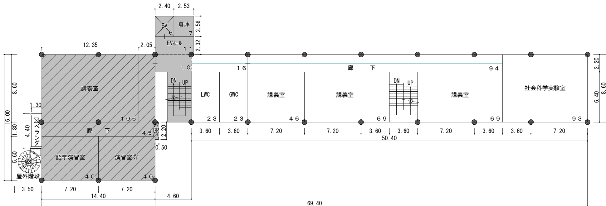
改修後 3階平面図 S=1/300
