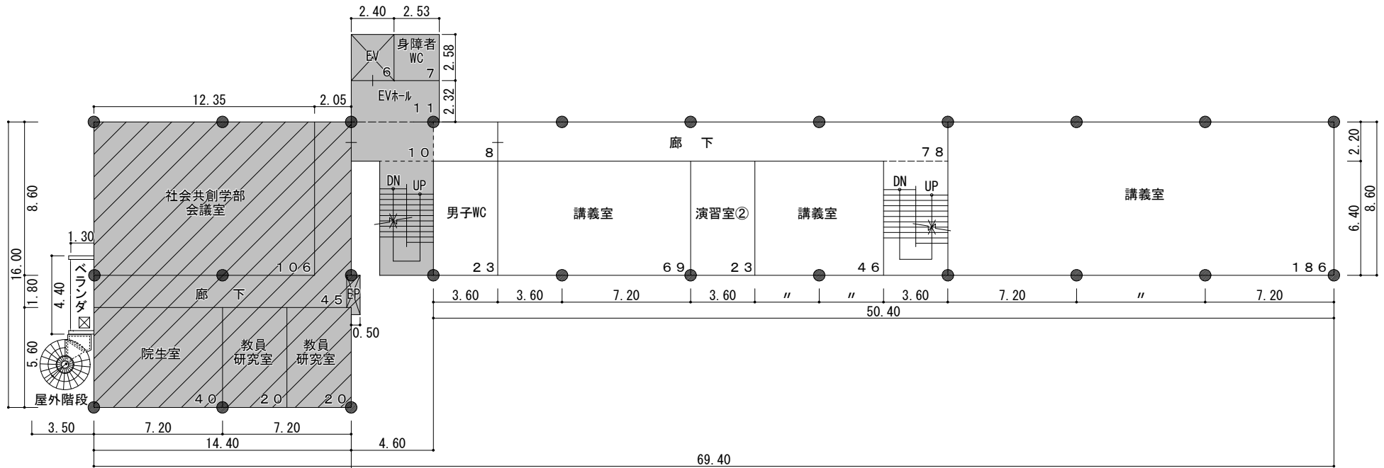
改修前 2階平面図 S=1/300
