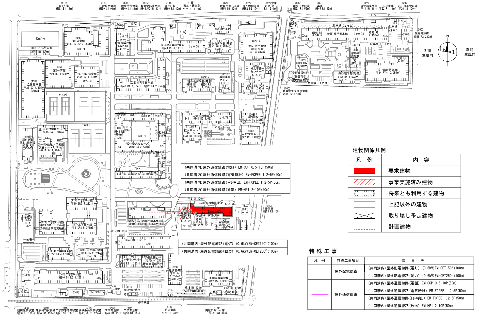
城北団地 配置図 S=1/2,500
