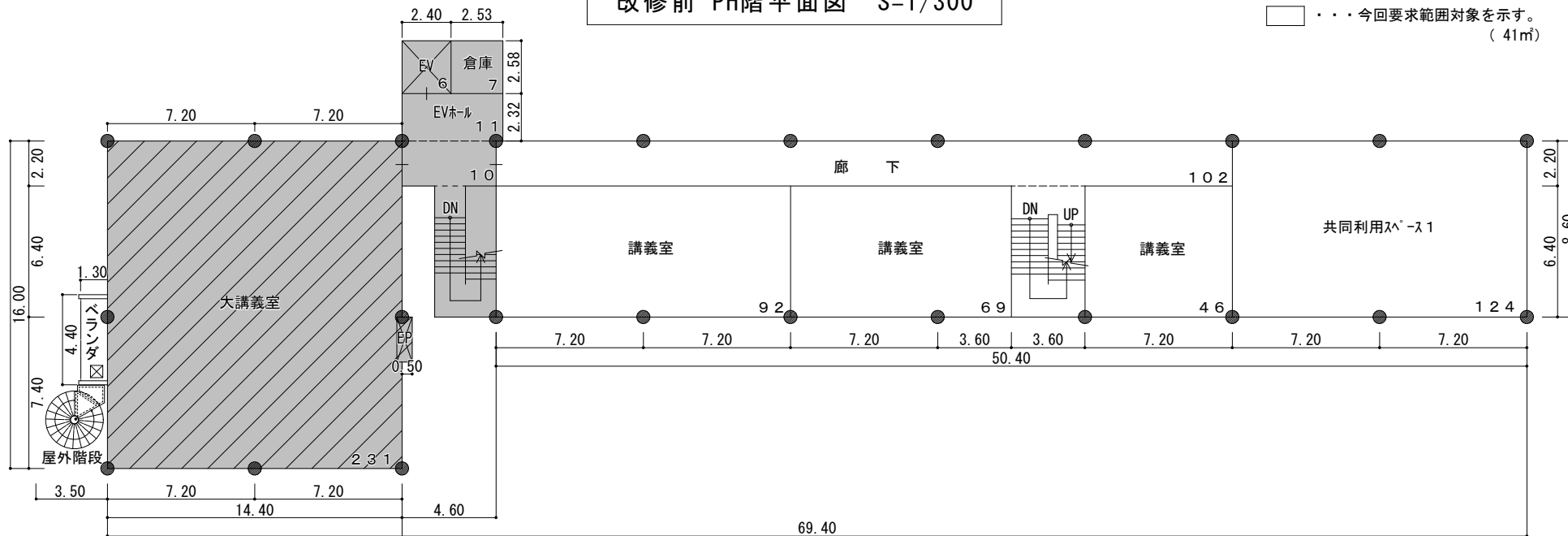
改修前 4階平面図 S=1/300
