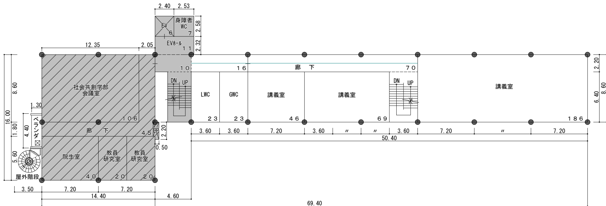
改修後 2階平面図 S=1/300
