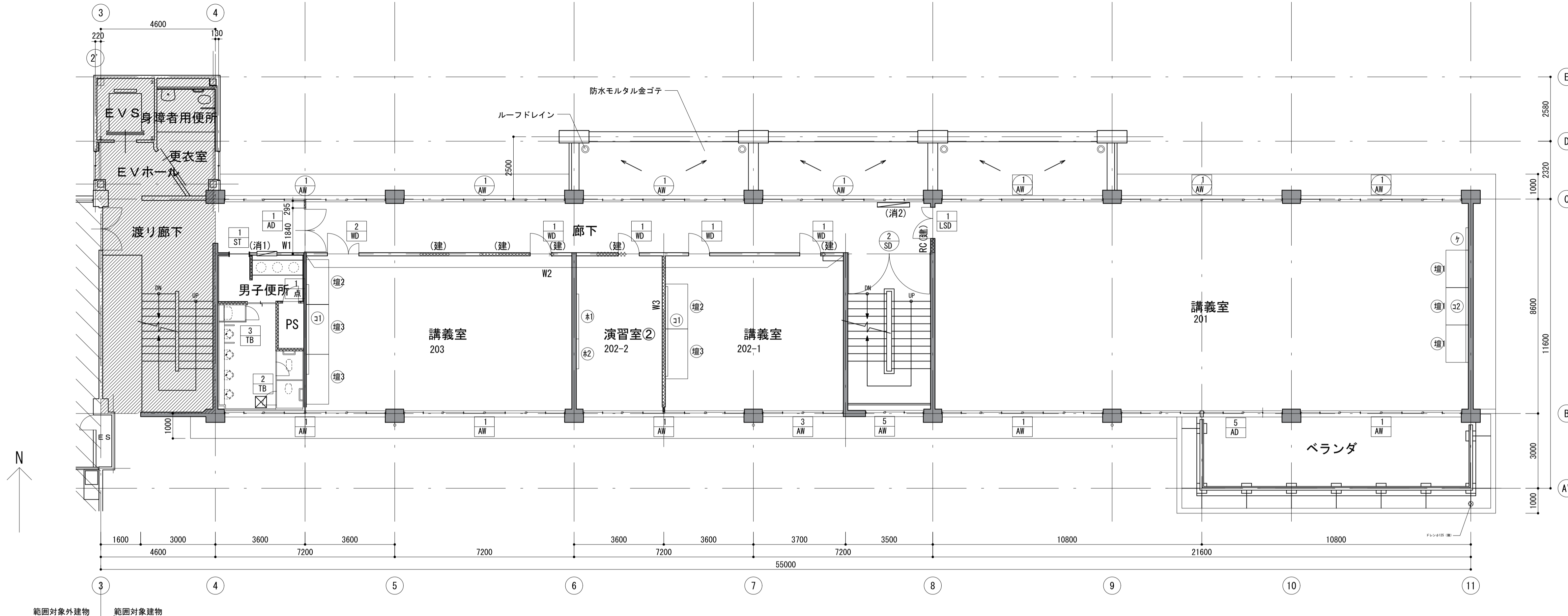
2階平面図(改修後)
