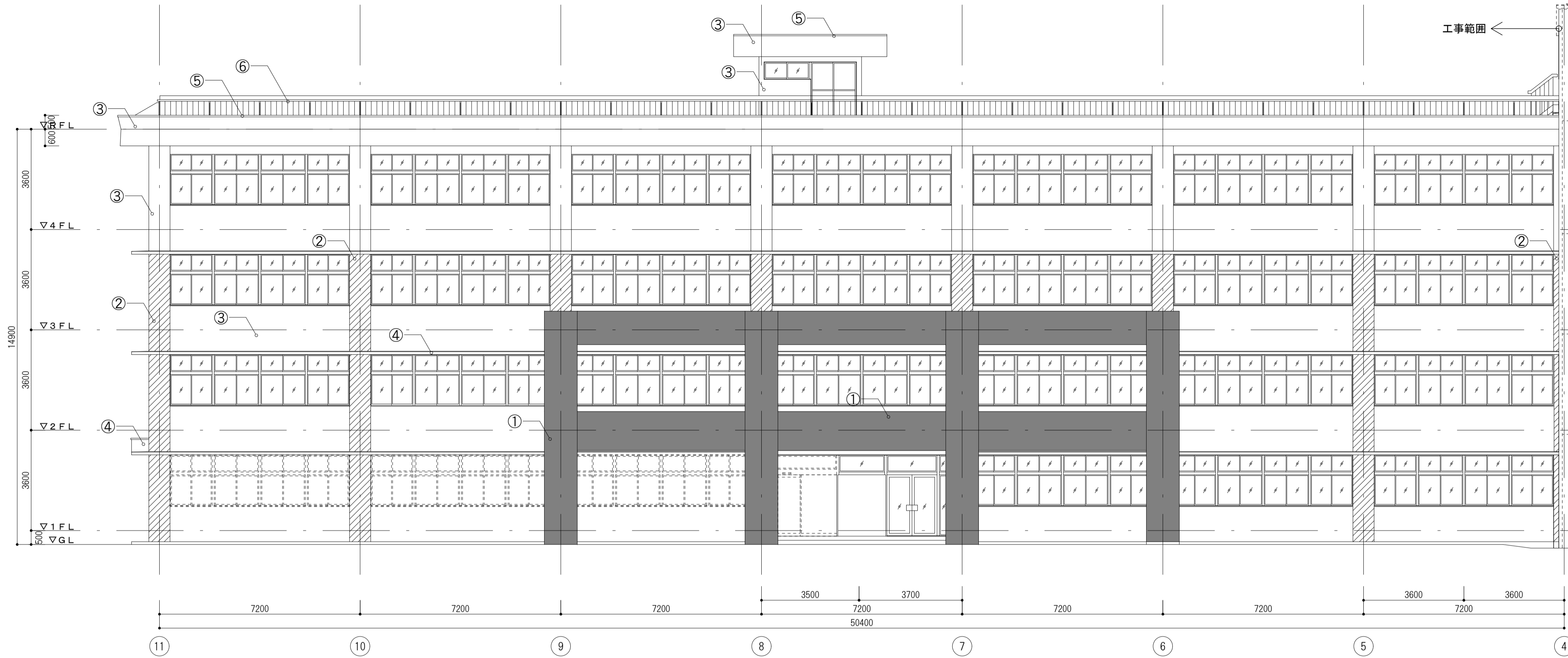
北側立面図
