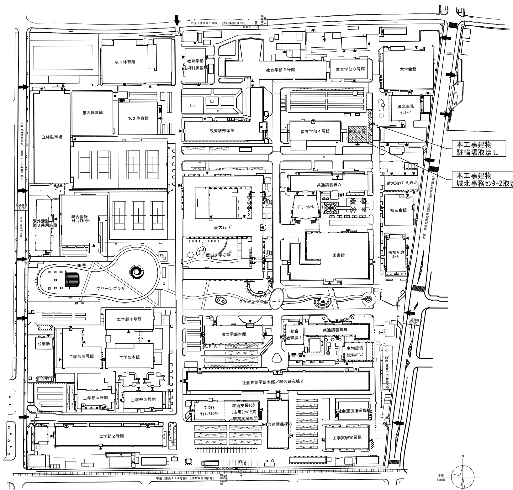
全体配置図 S=1/1,000
