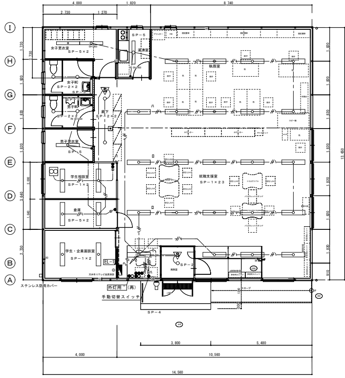
電灯配線撤去平面図 S=1/100 ※全て撤去とする。 ※LED照明器具については、大学へ引渡しとする。
