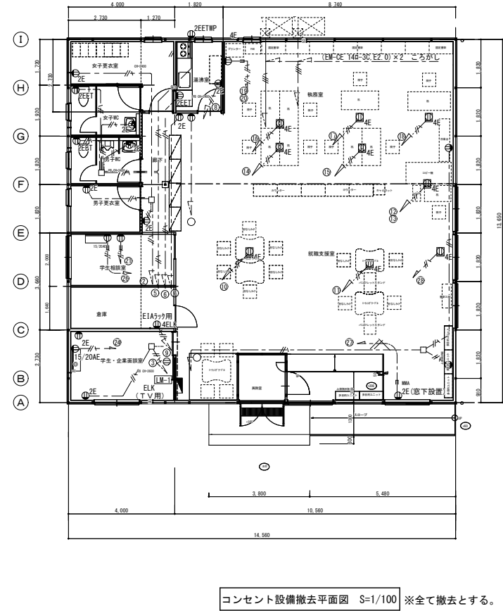
コンセント設備撤去平面図 S=1/100 ※全て撤去とする。
