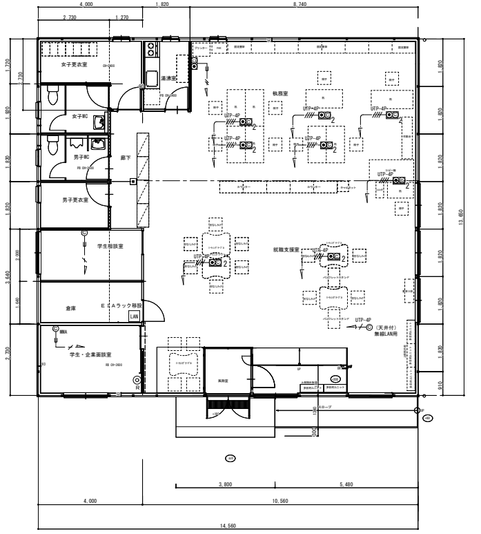
情報設備撤去平面図 S=1/100 ※全て撤去とする。
