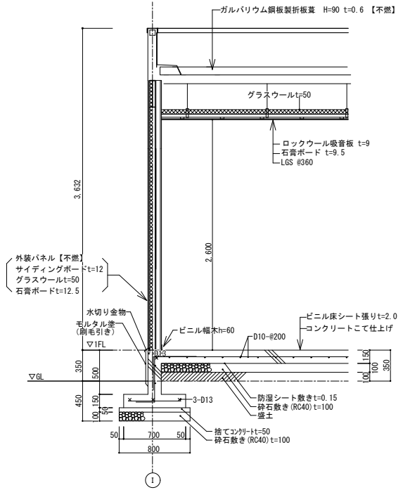
断面図 S=1/100
