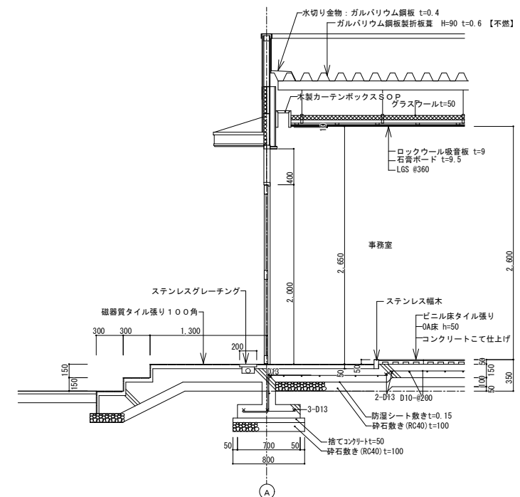
矩計図 (1) S=1/30 ※全て撤去とする。
