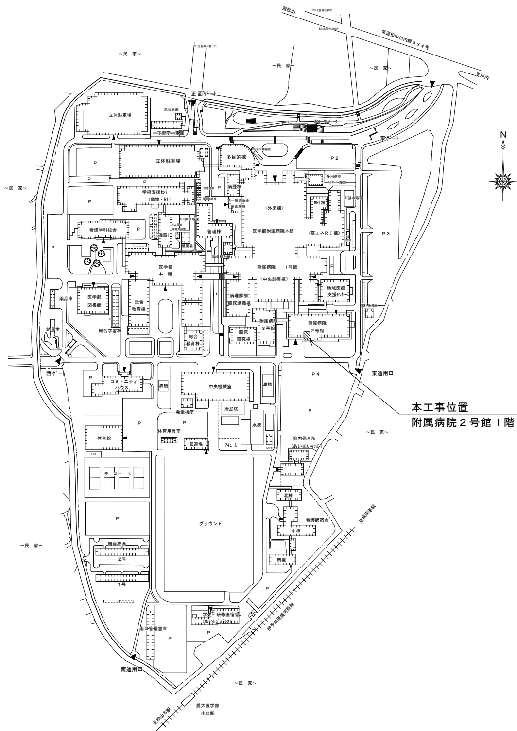
配置図 S=1/2000
