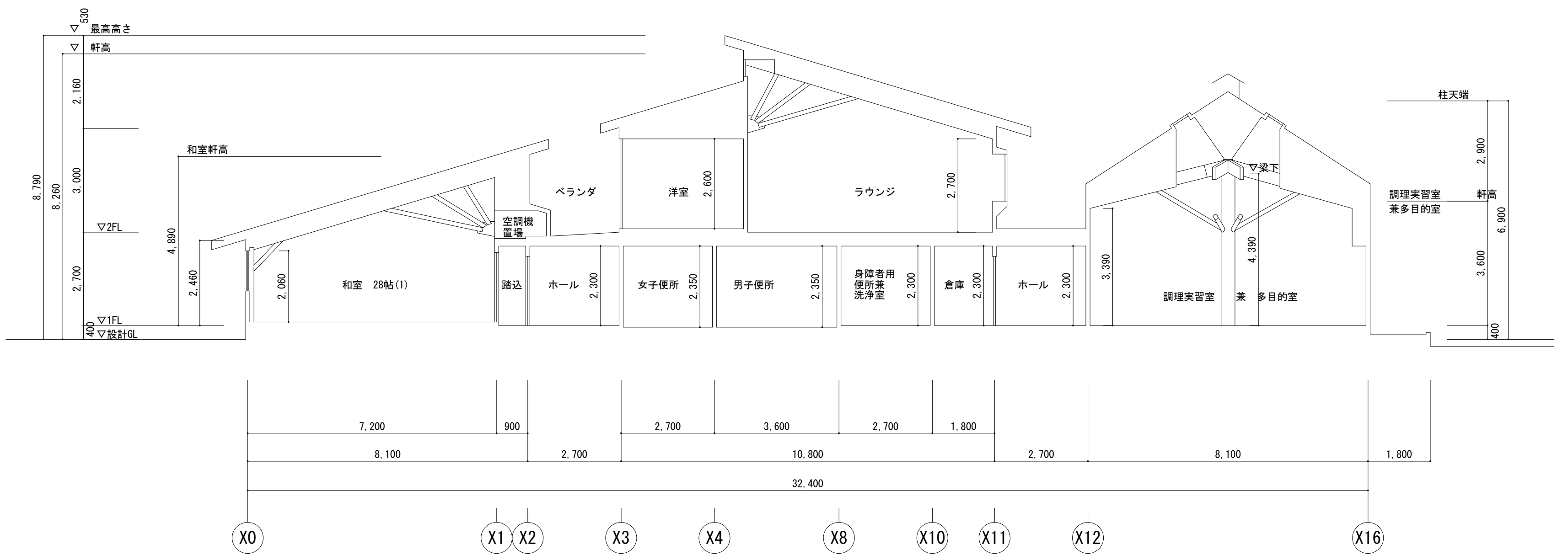
A-A' 断面図 S=1/100
