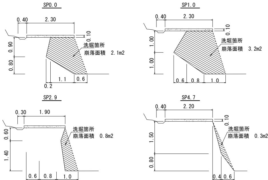
現況横断面図 (岩屋小屋林道) S=1/50
