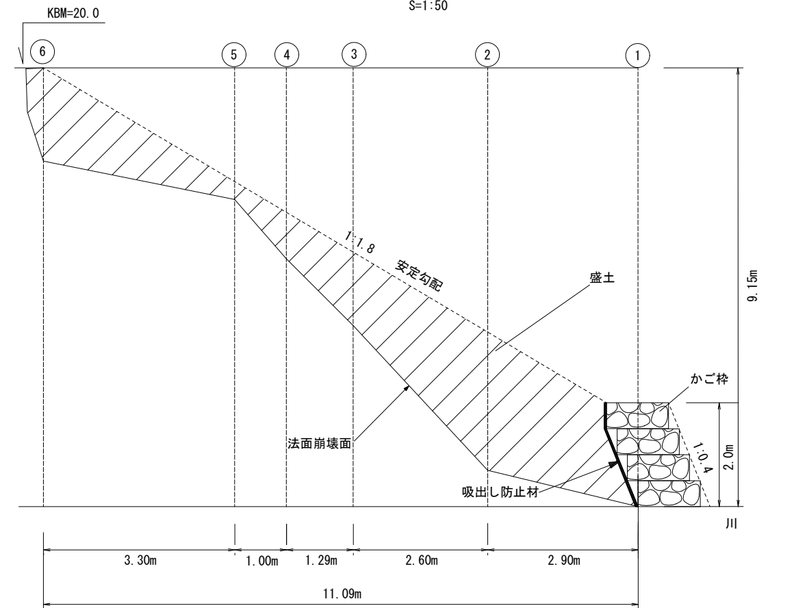
復旧横断面②
