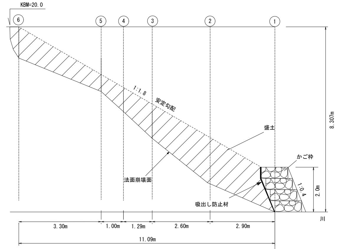
復旧横断面②
