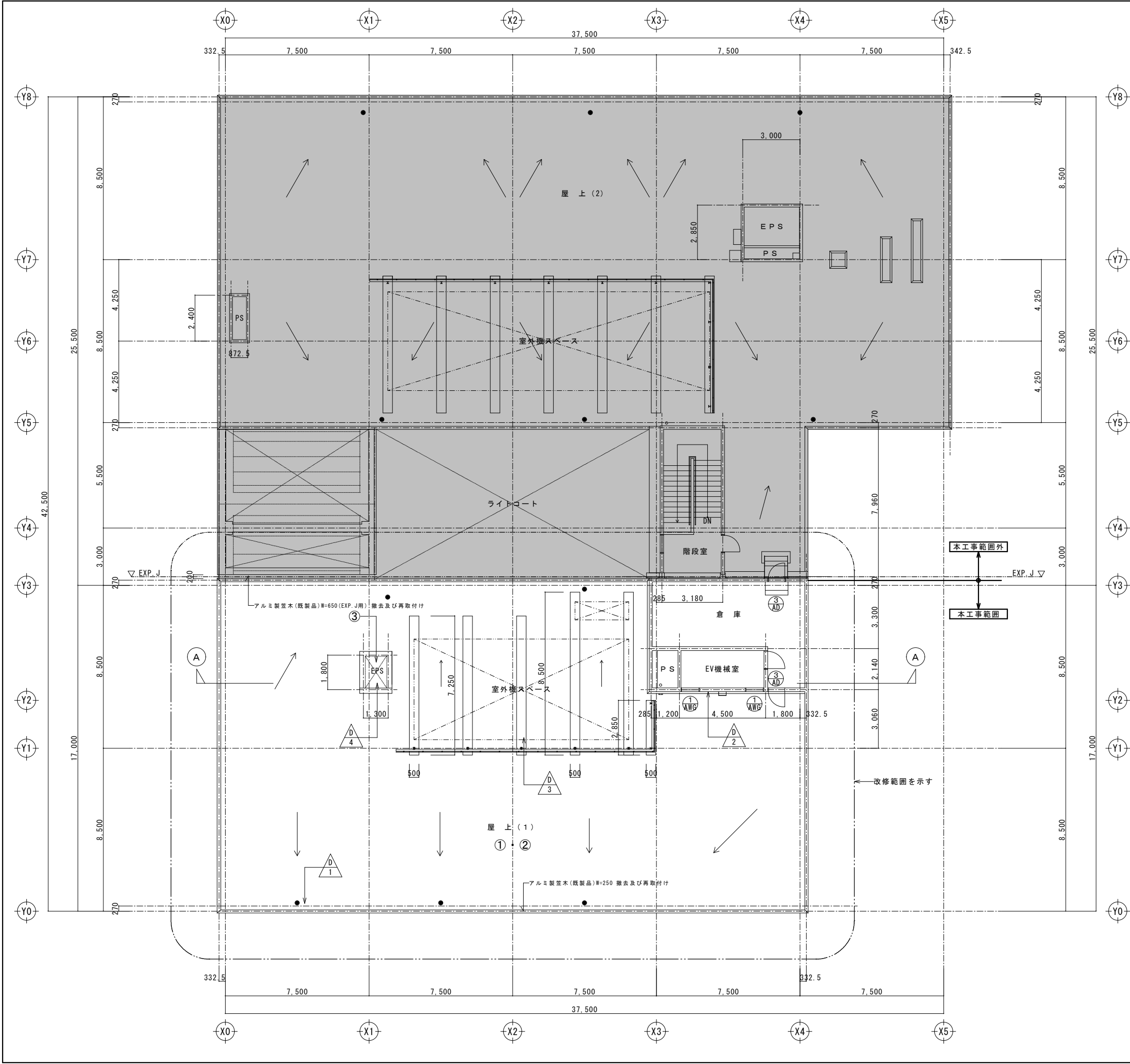
R 階平面図 S=1/100
