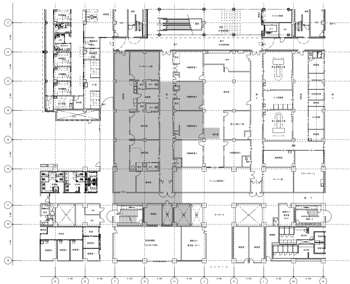
本館1階 平面図 S=1/200
