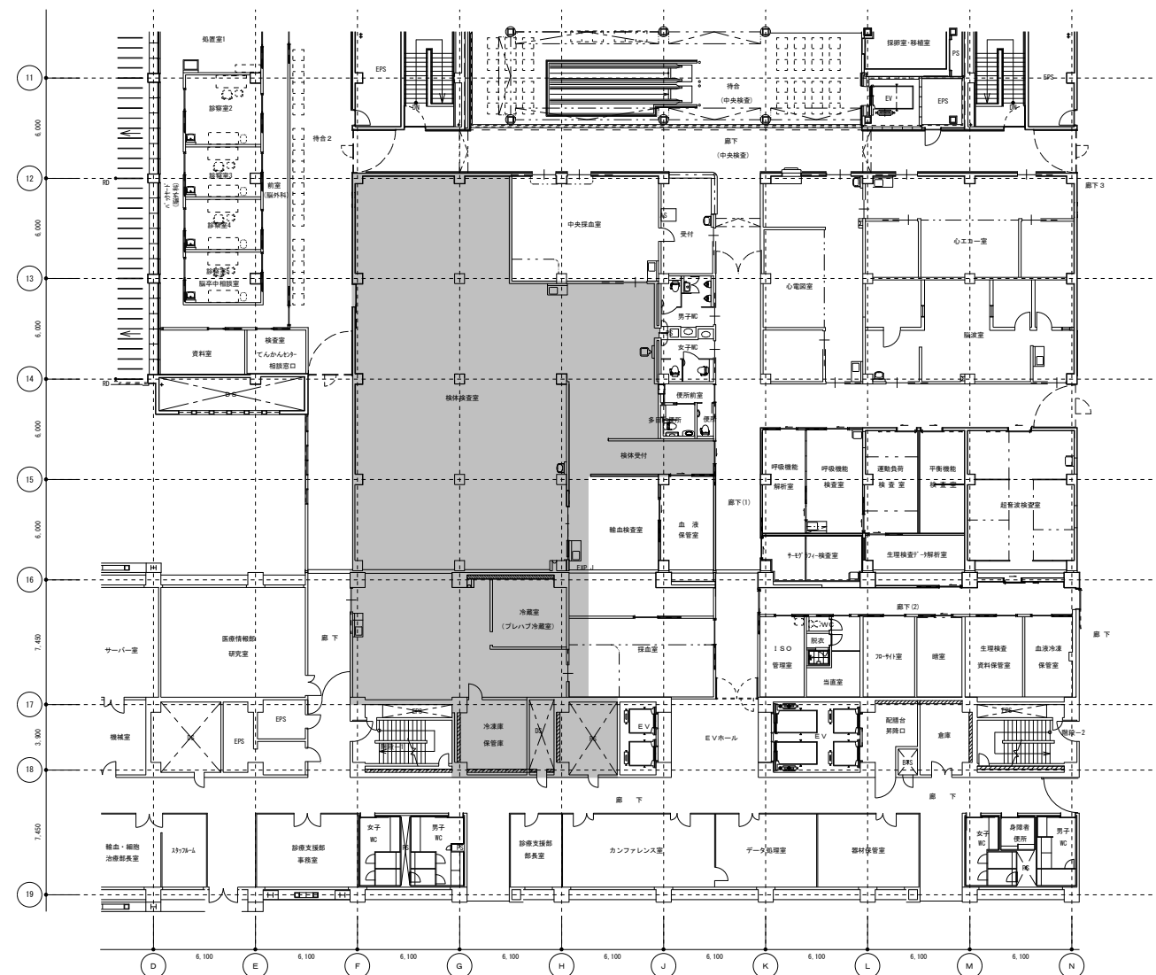
本館2階 平面図 S=1/200
