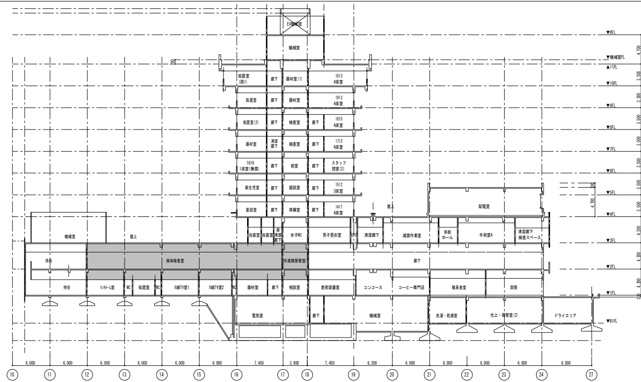
本館A-A' 断面図 S=1/300
