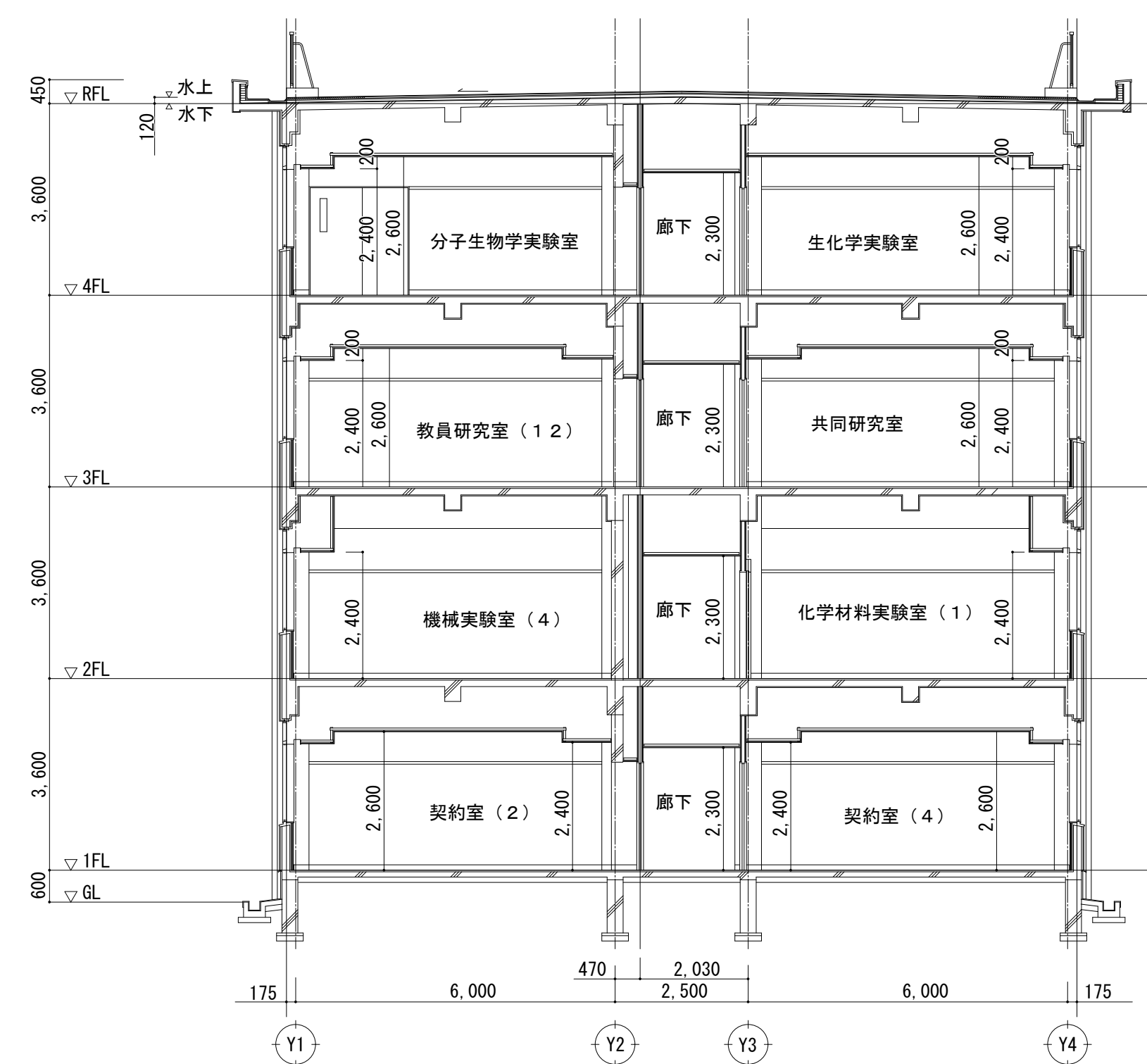
建物断面図 S=1/100
