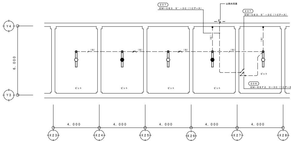
ビット階配線図 1:100
