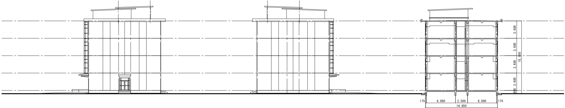
西側立面図
