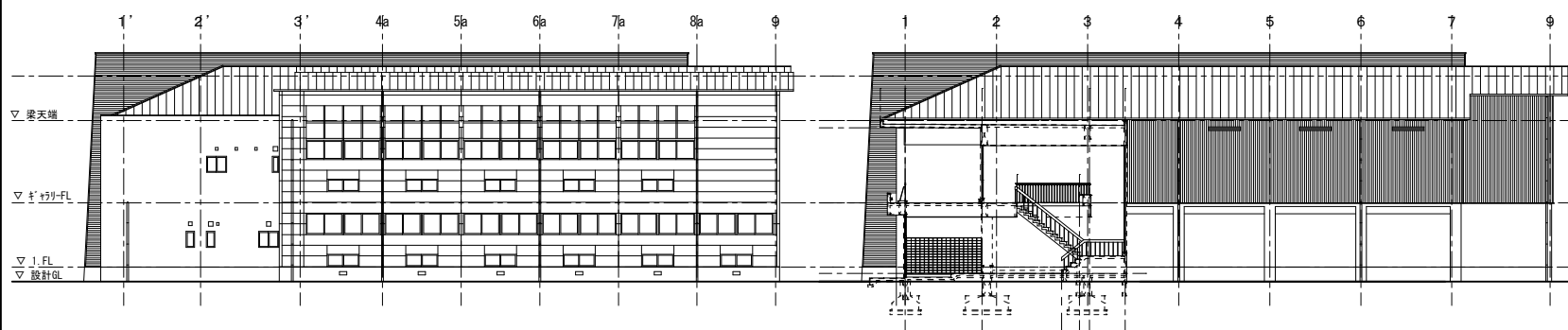
東立面図 A1 : S=1/200 A3 : S=1/400
