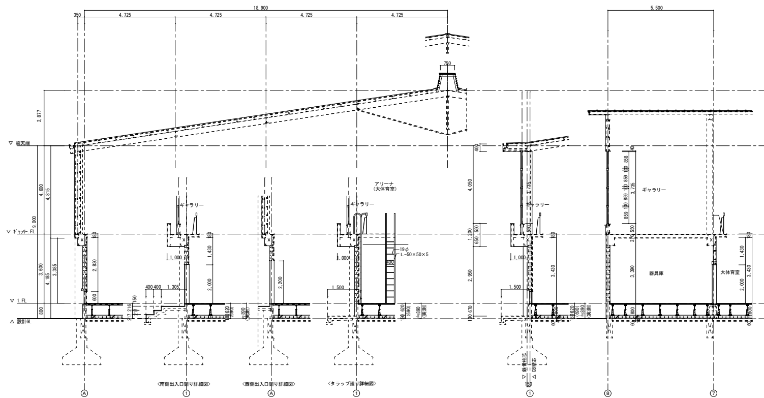
アリーナ断面図 A1 : S=1/100 A3 : S=1/200
