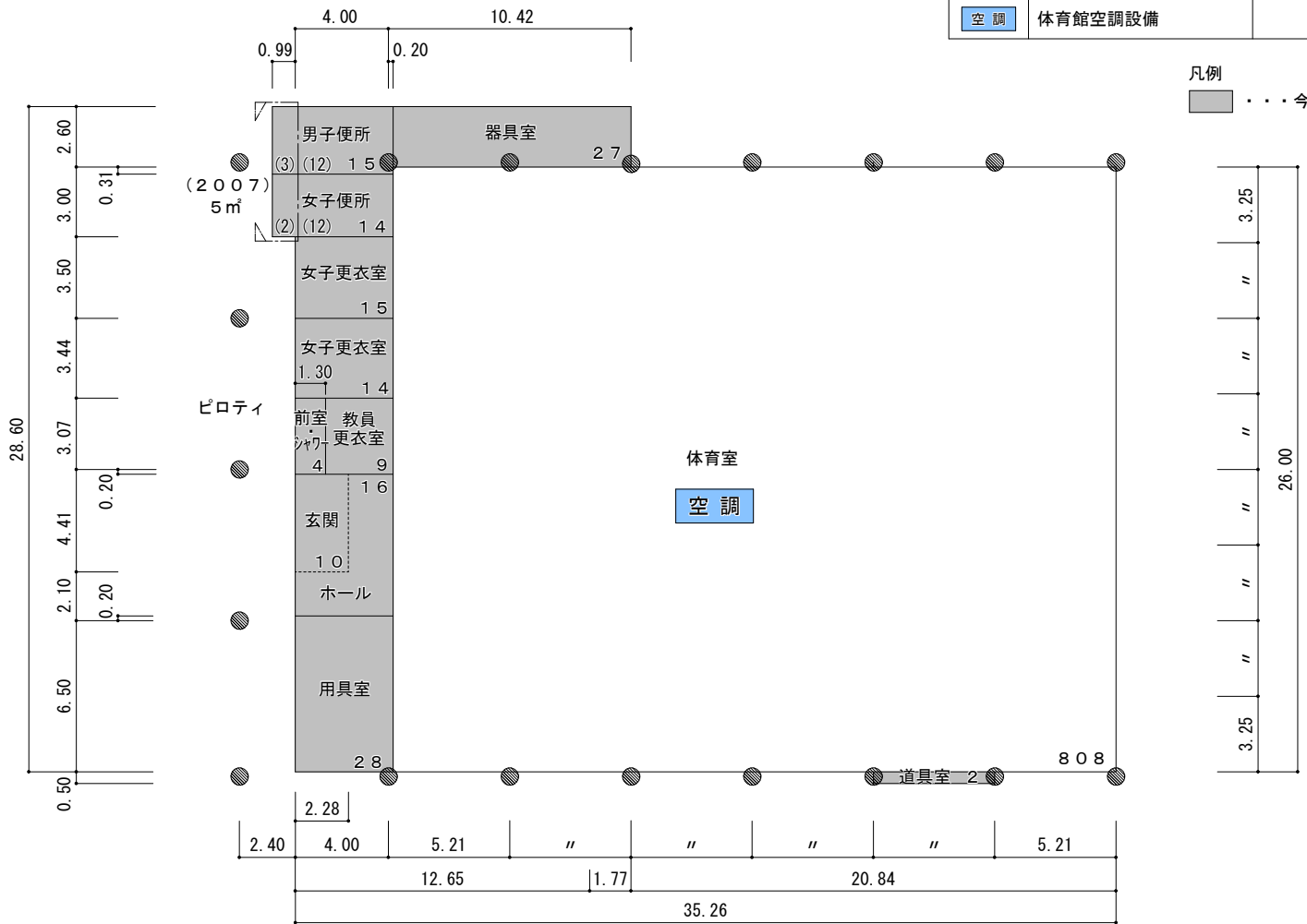
(003) 附属中学校体育館 1 階平面図 S=1/300 床面積 902㎡
