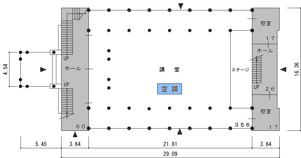
(001) 講堂 1 階平面図 S=1/300 床面積 476㎡
