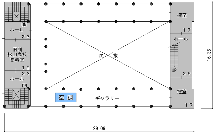
(001) 講堂 2 階平面図 S=1/300 床面積 125㎡
