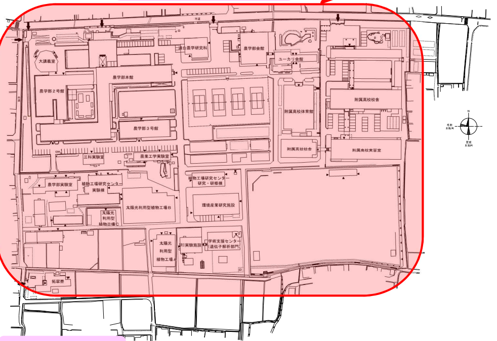
樽味団地配置図
